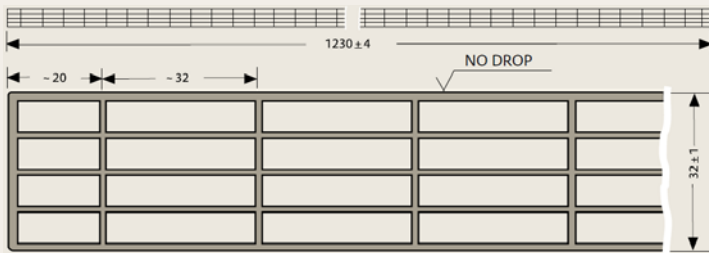
Querschnitt der PLEXIGLAS® Heatstop Opal S5P 32 (Maße in mm)
